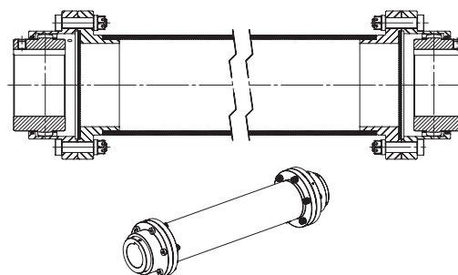
Esecuzione speciale con albero intermedio
